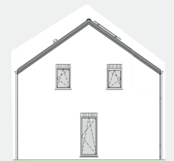
Pignon gauche
